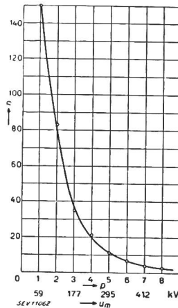
Fig. 4. Häufigkeitskurve der an der 80-kV-Leitung in Lavorgo im Sommer 1937 mit Klydonographen gemessenen absoluten Ueberspannungen
