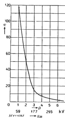
Fig. 5. Häufigkeitskurve der an der 80-kV-Leitung in Bodio im Sommer 1937 mit Klydonographen gemessenen absoluten Ueberspannungen
