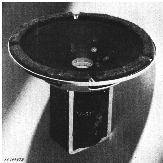
Fig. 1. Dynamischer Wandler
