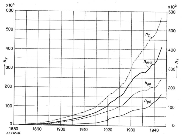
Fig. 11. Trafic téléphonique 1882...1943
