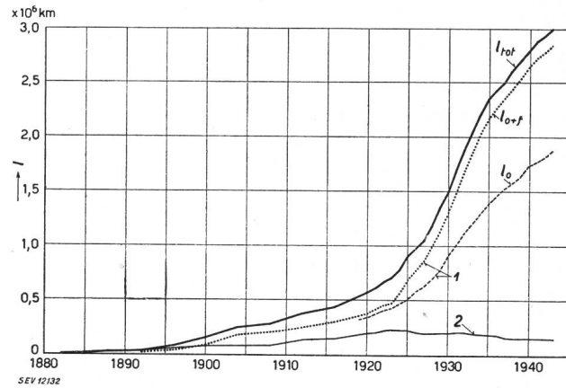
Fig. 9. Longueurs de fils du réseau téléphonique 1882...1943
