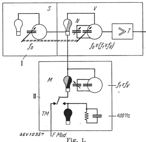
Schema eines Empfänger-Prüfsenders mit HF-Modulationszusatz zur Bandbreitenmessung
