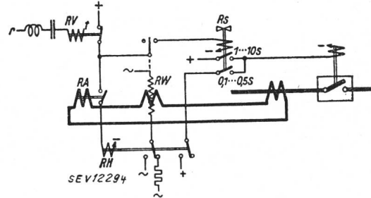
Fig. 5. Einpolig dargestellte Entkopplungseinrichtung RV Spannungsrelais. RA Stromrelais. RW Richtungsrelais. RS Zeitrelais. RH Hilfsrelais.
