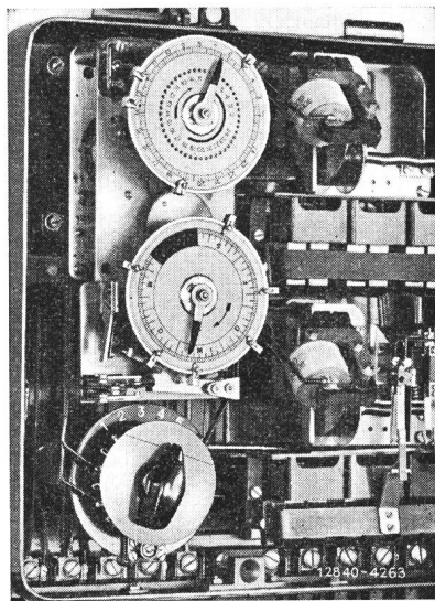
Fig. 3. Teilansicht eines Spezialzeitschalters mit Tages- und Wochenprogramm Obere Scheibe: Tagesprogramm; Untere Scheibe: Wochenprogramm; Darunter: Wahlschalter für beliebige Kombination der beiden Programmschaltungen.
