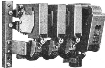
Fig. 2. Luftschütze 500 V, 100 A mit magnetischer Funkenlöschung und angebaute Signalwechsler
