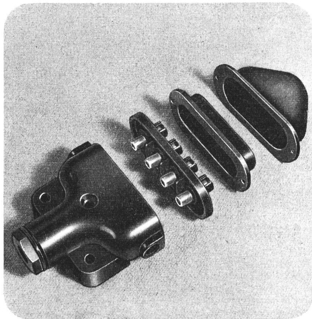
Fig. 2. Kabelendverschluss
