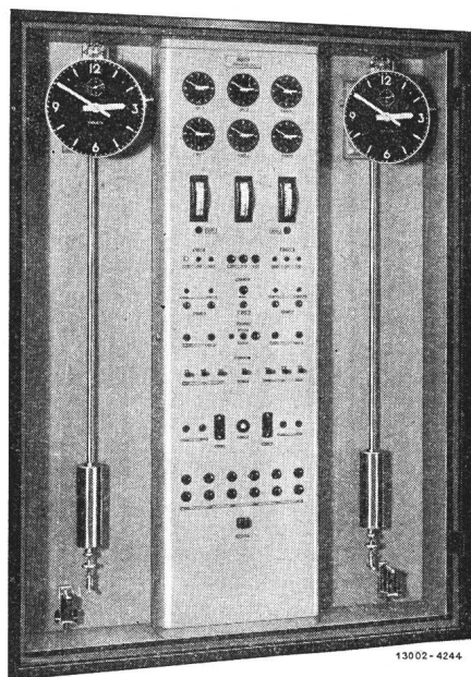
Fig. 4. Zeituhrenzentrale «Inducta» für die Steuerung einer grossen Anzahl von Nebenuhren in einem Industriebetrieb
