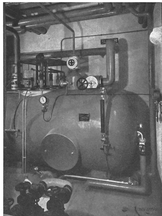
Fig. 5. Elektrokessel, liegende Form, max. Leistung 600 kW 1000 V; 16 \frac{2}{3} Hz.
