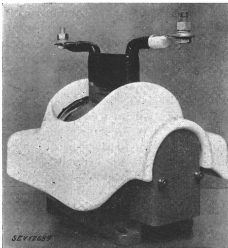
Fig. 9. Trockenstromwandler, Querlochtyp
