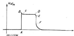
Fig. 6. SEV 12556 Steuerspannungsverlauf bei brennender Anode
