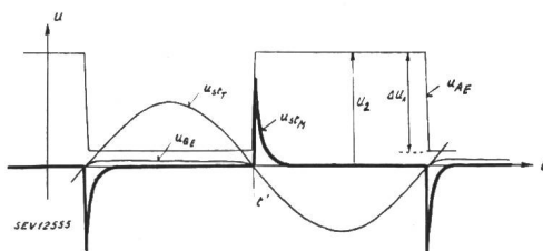
Fig. 5. Verlauf der Spannungen im Elektronenröhren-Steuergerät (Spannungen auf das Potential der Elektronenröhrenkathode bezogen)
