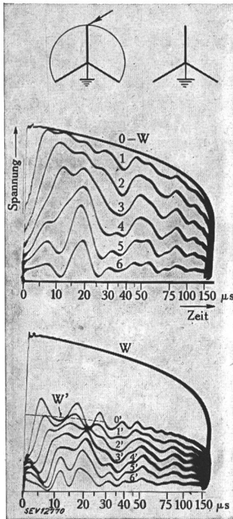
Fig. 1. Oscillogrammes des tensions dans les enroulements d'un transformateur soumis à une tension de choc primaire 0,0' tension aux bornes 1, 2, 3, 4, 5, 6 tension de la fin de la première, 2me, 3me, 4me, 5me, 6me bobine de l'enroulement primaire, qui a reçu la tension de choc. b 1', 2', 3', 4', 5', 6' tension de la fin de la première, 2me, 3me, 4me, 5me, 6me bobine de l'enroulement secondaire. W tension de choc primaire. W' tension de choc primaire réduite au secondaire dans le rapport de transformation correspondant à la marche à vide du transformateur a couplage b tensions primaires c tensions secondaires (le secondaire ne débite pas)
