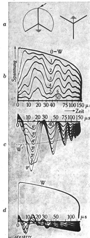
Fig. 2. Oscillogrammes des tensions dans les enroulements d'un transformateur soumis à une tension de choc primaire Légende: Voir fig. 1 a couplage b tensions primaires c tensions secondaires (le secondaire ne débite pas) d tensions secondaires (le secondaire débite sur une résistance de 500 \Omega par phase)
