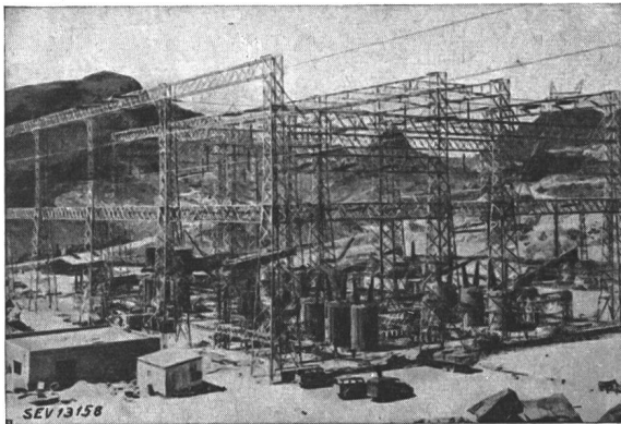
Fig. 21. Boulder Dam 287-kV-Freiluftanlage (Gerüsthöhe 35 m).
