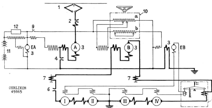
Verschiebelokomotive C-C der Französischen Staatsbahnen (SNCF) für den Dienst am Ablaufberg
