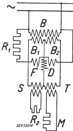
Fig. 3. Prinzipschema einer Wechselstrom-Brückenschaltung mit induktiven Zweigen B Brückentransformator B 1 , B 2 zwei Brücken-zweige, gebildet durch die Sekundärwicklung von B D Drehspule } des Anzeige-instruments F Feldwicklung } T Isoliertransformator M Messelement (variabler Widerstand) S Vergleichstransformator R 2 Konstanter Widerstand S, T bilden die übrigen beiden induktiven Brücken-zweige.
