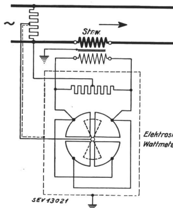
Bürdenmesser für Strom- und Spannungswandlerbürden
