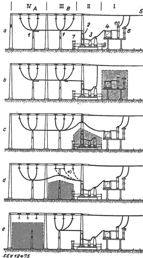
Fig. 4. Ueberbrückungsmöglichkeiten ausgefallener Geräte bei der Kiellinie
