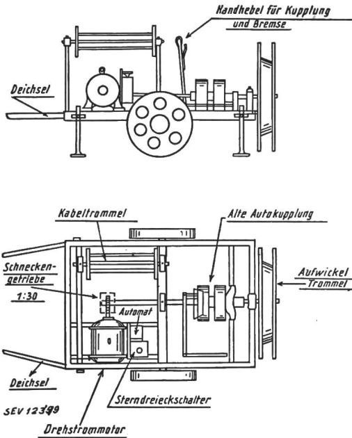
Fig. 1. Elektrisch angetriebene Seilwinde für das Abziehen von Leitungssellen
