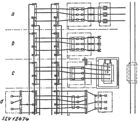
Fig. 3. Kiellinienbauweise, Stand 1942, in portalloser Rohrleiterausführung
