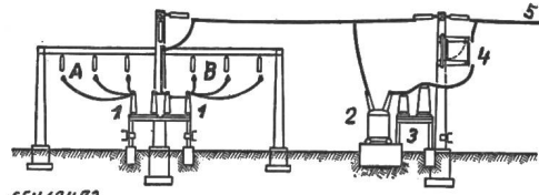
Fig. 2. Halbhohe Mittelmastbauweise
