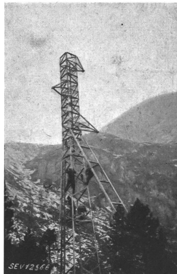
Fig. 6. Umgebauter Gittermast
