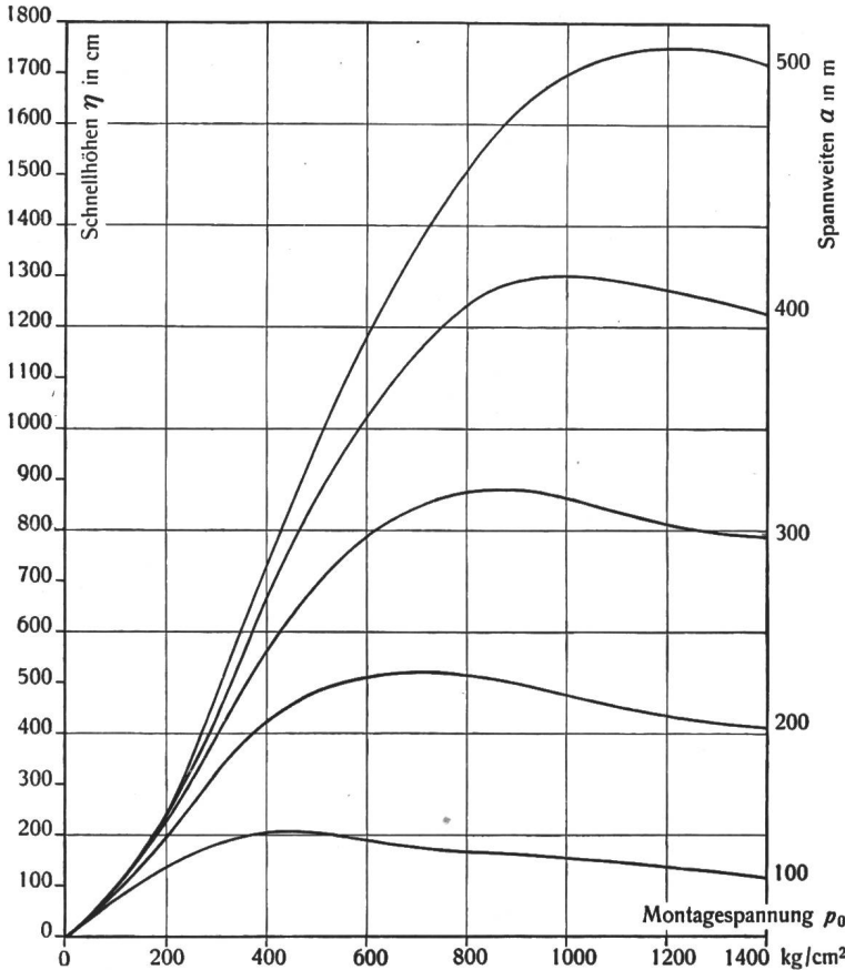
Fig. 3. Schnellhöhen η von 276-mm 2 -Aldrey-Seil in Abhängigkeit der Montagespannung p₀ für verschiedene Spannweiten a beim Abfallen einer Zusatzlast von 2 kg/m
