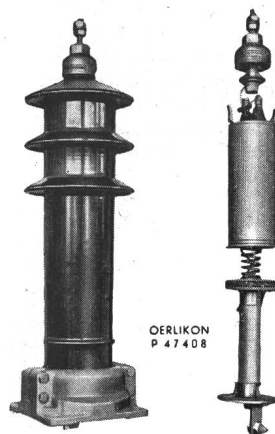
Fig. 4. Kondensator-Ueberspannungsableiter
