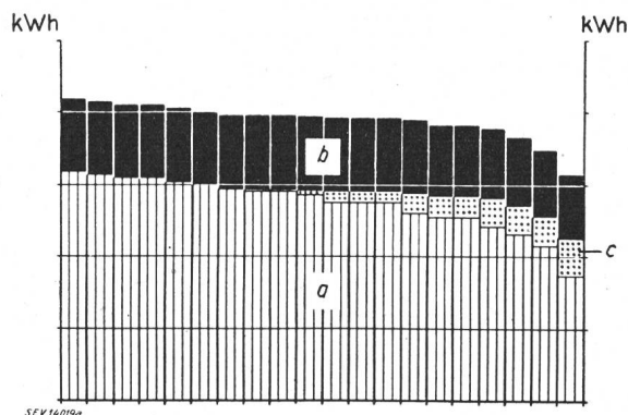
Fig. 8. Valorisation par l'énergie thermique de l'énergie des usines au fil de l'eau interconnectées avec des usines à accumulation (20 semestres d'hiver)
