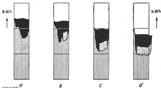
Fig. 7. Incorporation de la production thermique à la production combinée au fil de l'eau et à accumulation pour le semestre d'hiver
