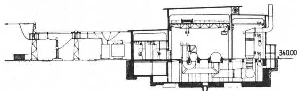
SEV 14017 0 10 20 m Station de transformation Salle des machines
