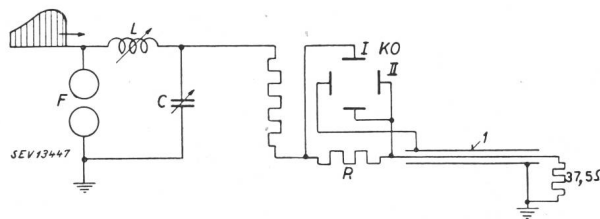
Fig. 7. Schaltung zur Messung des Phasenwinkels des Wellenwiderstandes i Verzögerungskabel
