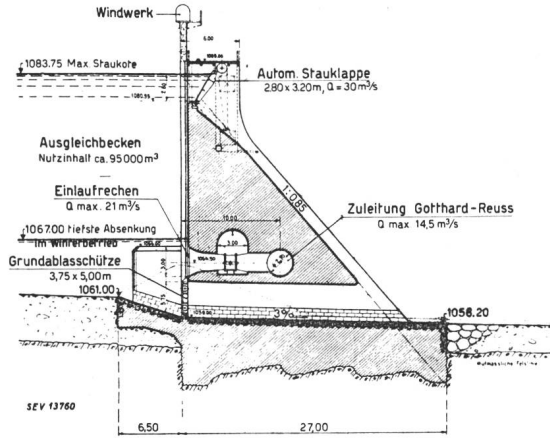
Fig. 4. Kraftwerk Wassen, Wasserfassung Göschenen, Schnitt durch die Staumauer
