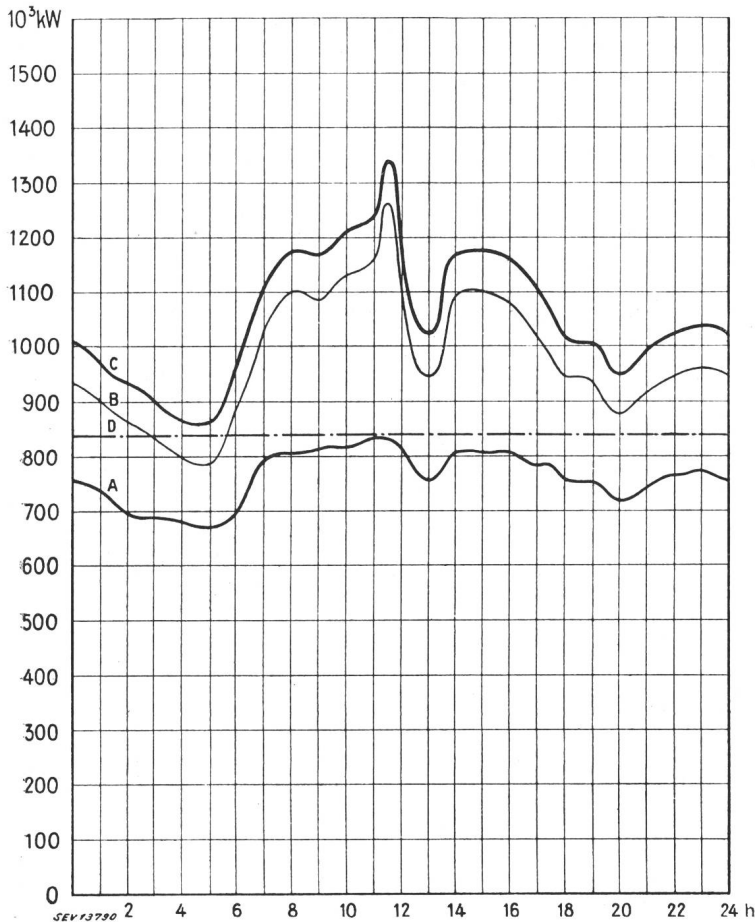
Diagramme de charge journalier du mercredi 12 juin 1946
