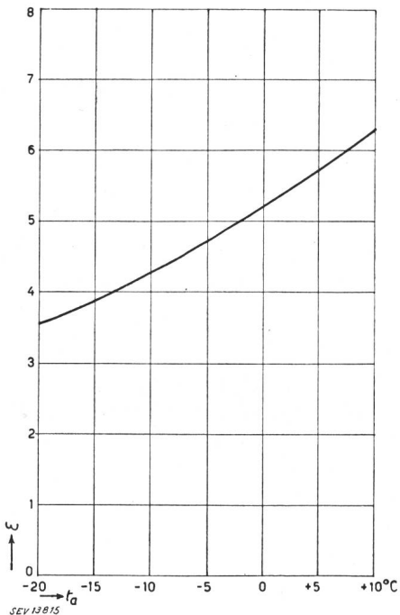
Fig. 5. Leistungsziffern \varepsilon in Abhängigkeit der Aussentemperaturen t_a (auf Grund von Fig. 4)
