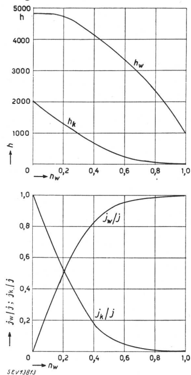
Fig. 3. Graphische Darstellung der jährlichen Benützungsdauern h_w, h_k und der Verhältnissfaktoren j_w/j, j_k/j in Funktion des Leistungsanteils der Wärmepumpe n_w
