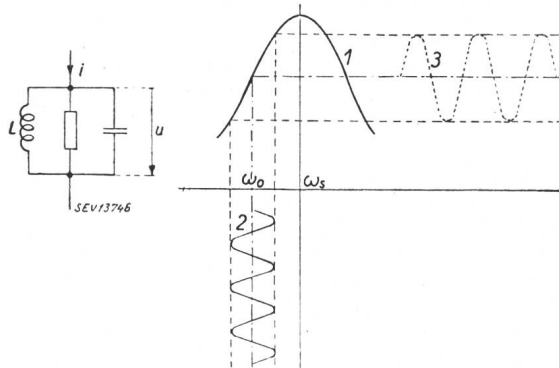
Fig. 2. Resonanzkreis-Diskriminator
