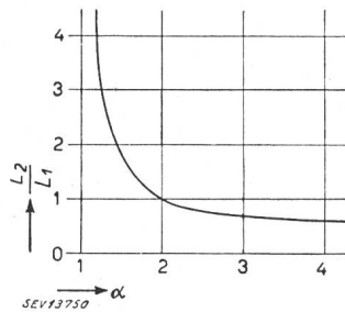
Fig. 6. Charakteristik der Funktion \frac{L_2}{L_1} = f(\alpha) für den Spezialfall Q_1 = Q_2 = Q
