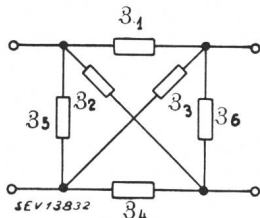
Schaltung des allgemeinsten passiven Vierpols
