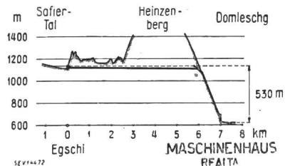
Fig. 1 Kraftwerk Rabiusa-Realta Längenprofil
