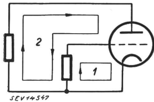
Fig. 1 Prinzipialschaltung eines Röhrenverstärkers 1 Gitterkreis, 2 Anodenkreis
