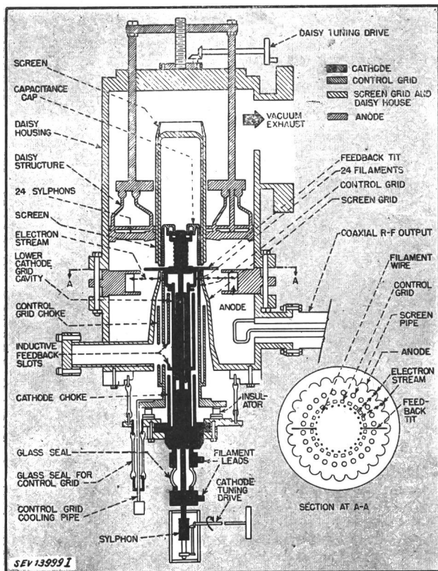
Fig. 8 Schnitt durch ein Resatron Betriebswellenlänge \lambda = 50 cm, Dauerleistung 50 kW
