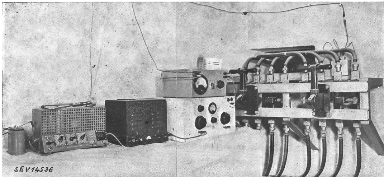
Fig 1 Netzrundspruch-Versuchsanlage (Airolo)
