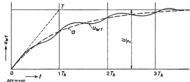
Fig. 4 Zeitlicher Verlauf der Windungsspannung der ersten Windung (für den Fall T/T k = 1) u w1 Windungsspannung; a Exponentialkurve des mittleren Spannungsanstiegs; U angelegte Stoßspannung; T Zeitkonstante; T k Eigenschwingungsperiode; t Zeit.
