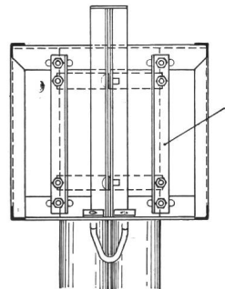
Fig. 9 Tragemast, Befestigung der Traverse an den Holzstangen Maßstab 1 : 25
