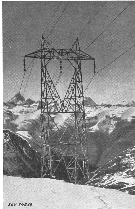
Fig. 4 Tragmast der Gebirgsstrecke bei der Nufenenpasshöhe mit Blick nach Norden (Berner Alpen)
