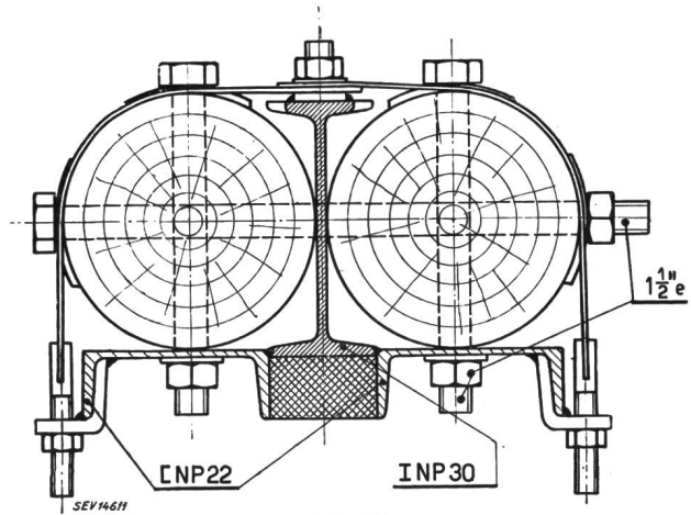
Fig. 14 Schnittzeichnung eines Sockels für Tragmasten Maßstab 1 : 10
