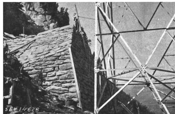
Fig. 31 «Grosse» Lawinenschutzmauer eines Tragemastes
