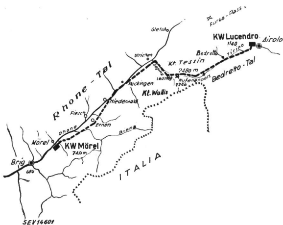
Fig. 1 150-kV-Leitung Mörel—Airolo, Situationsplan Maßstab 1 : 800 000
