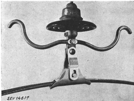
Fig. 19 Tragklemme AIAG
