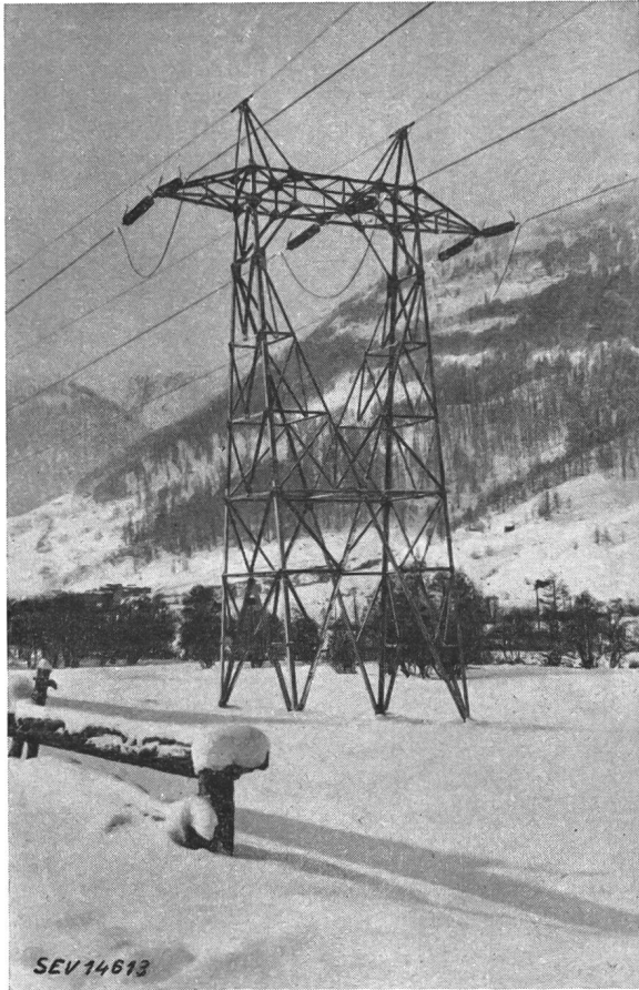
Fig. 3 Abspanneckmast der Talstrecke
