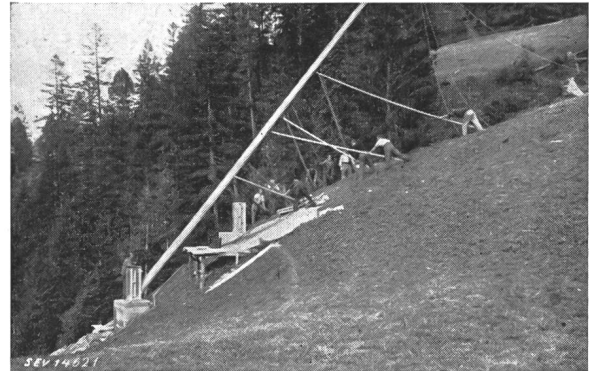
Fig. 23 Holztragmast mit Sockel, Stangenstellen
