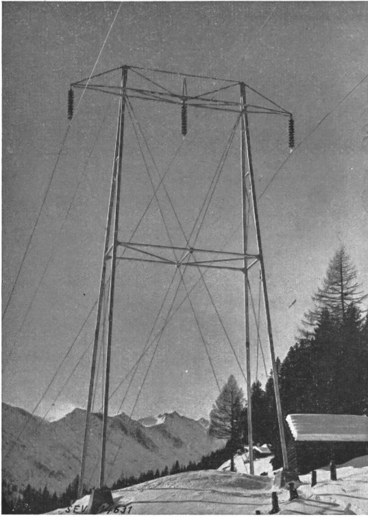
Fig. 5 Tragmast mit ausbetonierten Röhren der Talstrecke Bedretto
