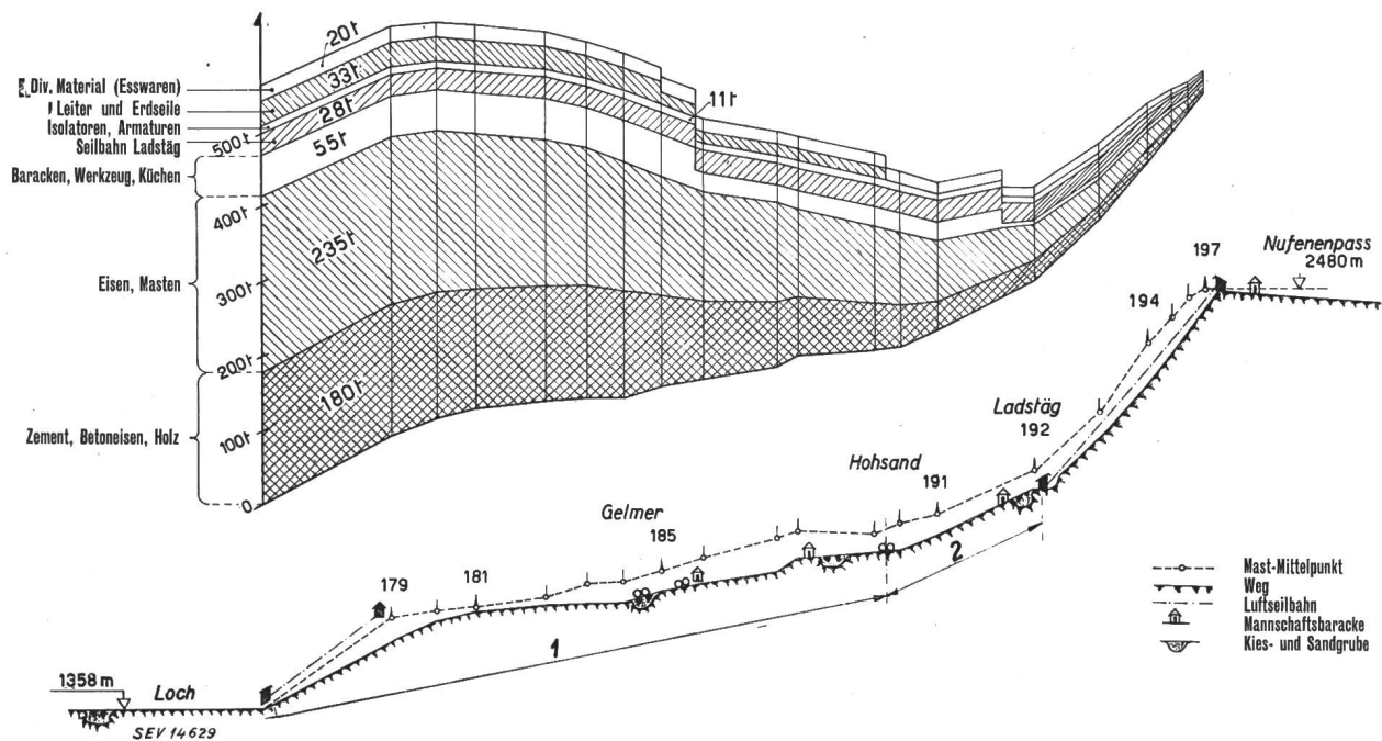
Fig. 28 Materialtransportgewichte der Gebirgstrecke (über Transportweg aufgetragen) 1 mit Traktor befahrbare Strecke; 2 Maulesel-Transport
