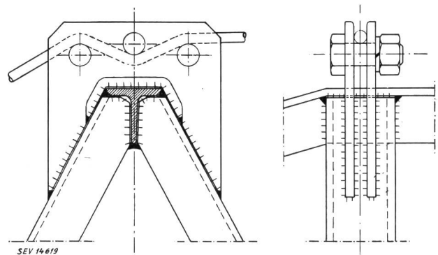
Fig. 21 Erdseilbefestigung bei Tragmasten Maßstab 1 : 5
