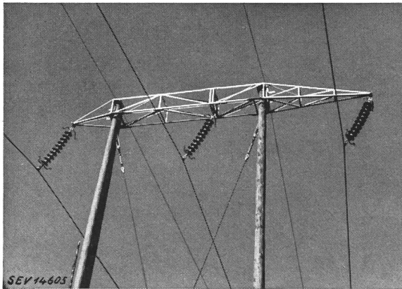
Fig. 8 Trageckmast, Oberteil
