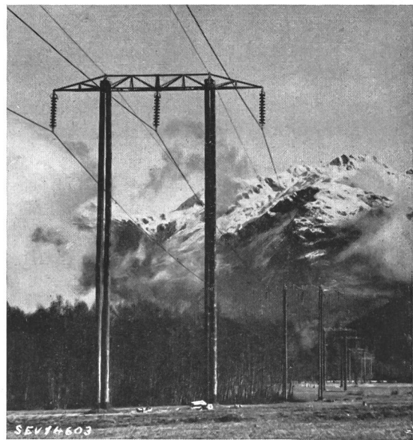
Fig. 6 Holztragmast mit 3 Reinaluminiumleitern von je 240 mm 2 und 2 Erdsellen von je 50 mm 2
