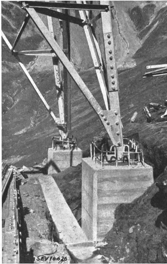
Fig. 29 Fundament vor Eingliessen, bzw. Aufbetonieren
