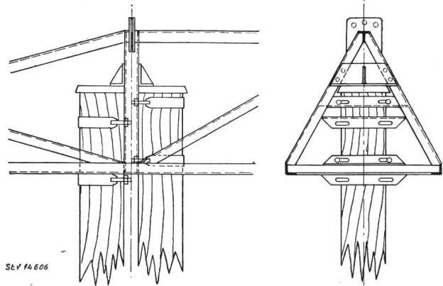
Fig. 9 Tragemast, Befestigung der Traverse an den Holzstangen Maßstab 1 : 25
