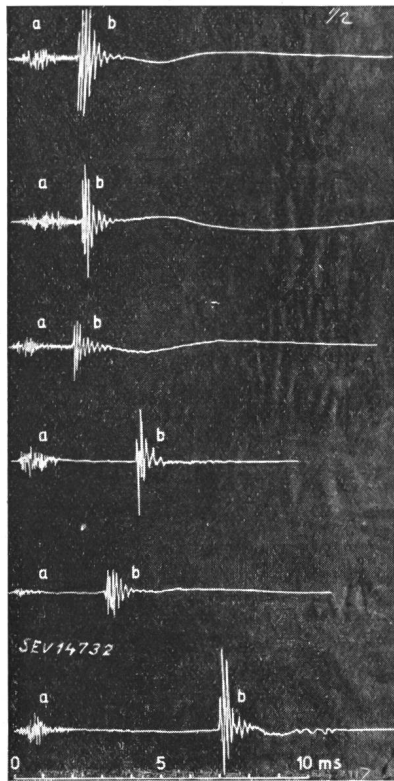
Fig. 11 Die Aufzeichnungen von Fig. 10 in deutlichem Zeitmaßstab a Vorentladung b Hauptentladung
