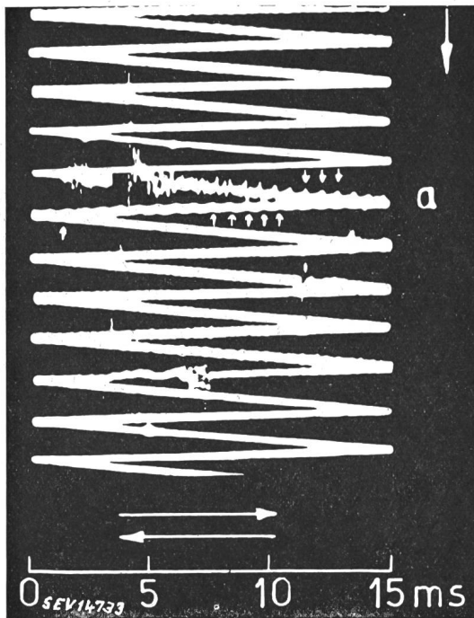
Fig. 12 Oszillogramme einer Blitzentladung mit typischer Vorentladung und Hauptentladung Die Pfeile markieren Reflexionen an der Ionosphäre
