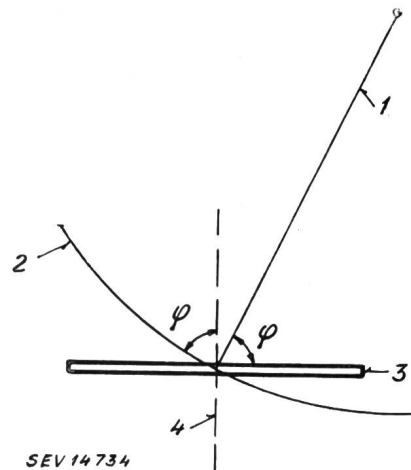
Fig. 13 Prinzip der Messungen mit der Rahmenantenne 1 Blitzbahn 2 Magnetfeldlinie 3 Rahmen 4 Rahmenachse
