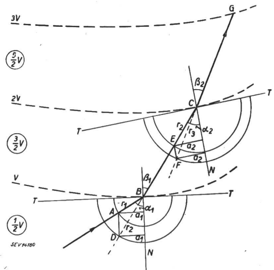
Fig. 2 Konstruktive Ermittlung der Brechungswinkel der Elektronenbahnen V, 2V, 3V Potentiallinien; \alpha_1, \alpha_2 Einfallswinkel; \beta_1, \beta_2 Austrittswinkel; N Normale zu den Potentiallinien; TT' Tangenten zu den Potentiallinien.
