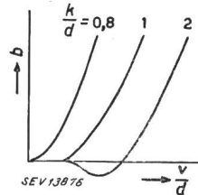
Fig. 3 Dämpfungskurven von Bandfiltern b Dämpfung des Bandfilters v relative Verstimung der Kreise d Dämpfung der Kreise k Kopplungsfaktor beider Kreise
