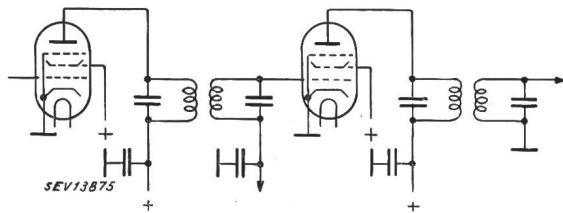
Fig. 2 Zwischenfrequenzverstärker eines Supers
