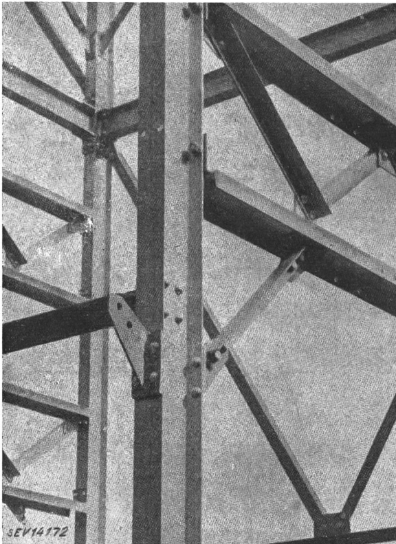
Fig. 4 Detail der Verschraubung und Nietung
