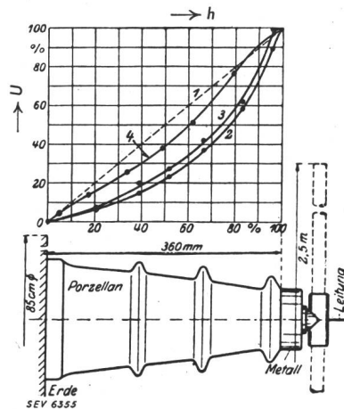
Fig. 6 Spannungsverteilung an der Aussenfläche eines parabolischen Stützers ohne Innelektroden bei Aufstellung auf geerdeter Platte 2 Die spannungsführende Leitung in der Verlängerung der Stützerachse 3 Die spannungsführende Leitung in parallel zur Erde 4 Der Isolator mit dem Kopf gegen Erde montiert
