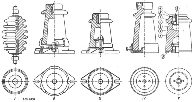
Fig. 1 Verschiedene Stützer-Bauarten
