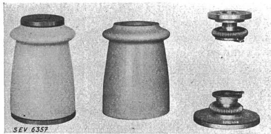
Fig. 2 Stützer Typ K Ansicht und Bestandteile
