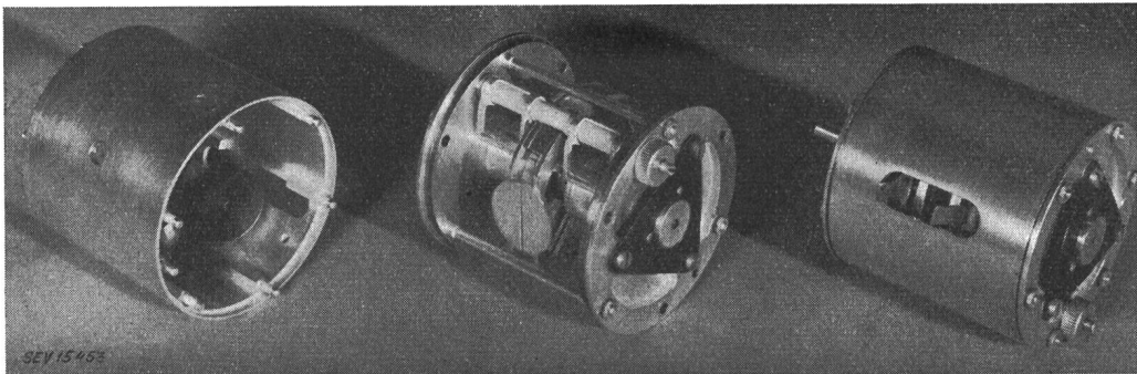
Fig. 11 Schwingtopf für Dezimeterwellen Schwingtopf-Resonatoren dieser Art wurden am Institut für Hochfrequenztechnik der ETH entwickelt
