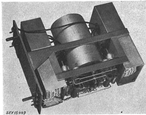
Fig. 7 Zweistufiges Kristallfilter
