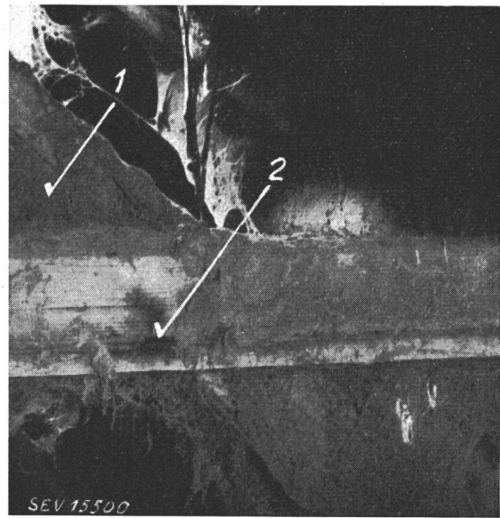
Fig. 5 Eine Schadenstelle der Isolierrohre 1 Schmutzschicht auf dem Balken der Firstzange 2 Schmelzspur an den armierten Isolierrohren (erst nach Entfernung der Spinnengewebe sichtbar geworden)
