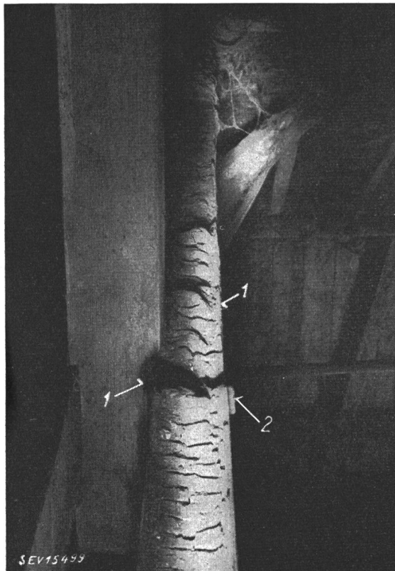
Fig. 4 Die Brandschäden an Stützbalken und Firstzange 1 angebrannte Balken der Firstzange 2 Verbindungsschraube
