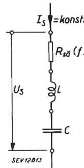
Fig 8 Die wirkleistungsmässig der Schaltung Fig. 7 äquivalente Seriekreis-schaltung mit konstantem Strom (2. Fall) Der äquivalente Seriewiderstand ist trotz Frequenzabhängigkeit rein ohmisch zu denken
