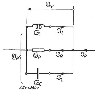
Fig. 2 Reine Parallelschaltung
