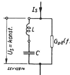
Fig. 9 Die wirkleistungsmässig der Schaltung Fig. 7 äquivalente Seriekreis-schaltung mit konstanter Spannung (1. Fall) Der äquivalente Parallel-Leiter ist trotz Frequenzabhängigkeit rein ohmisch zu denken
