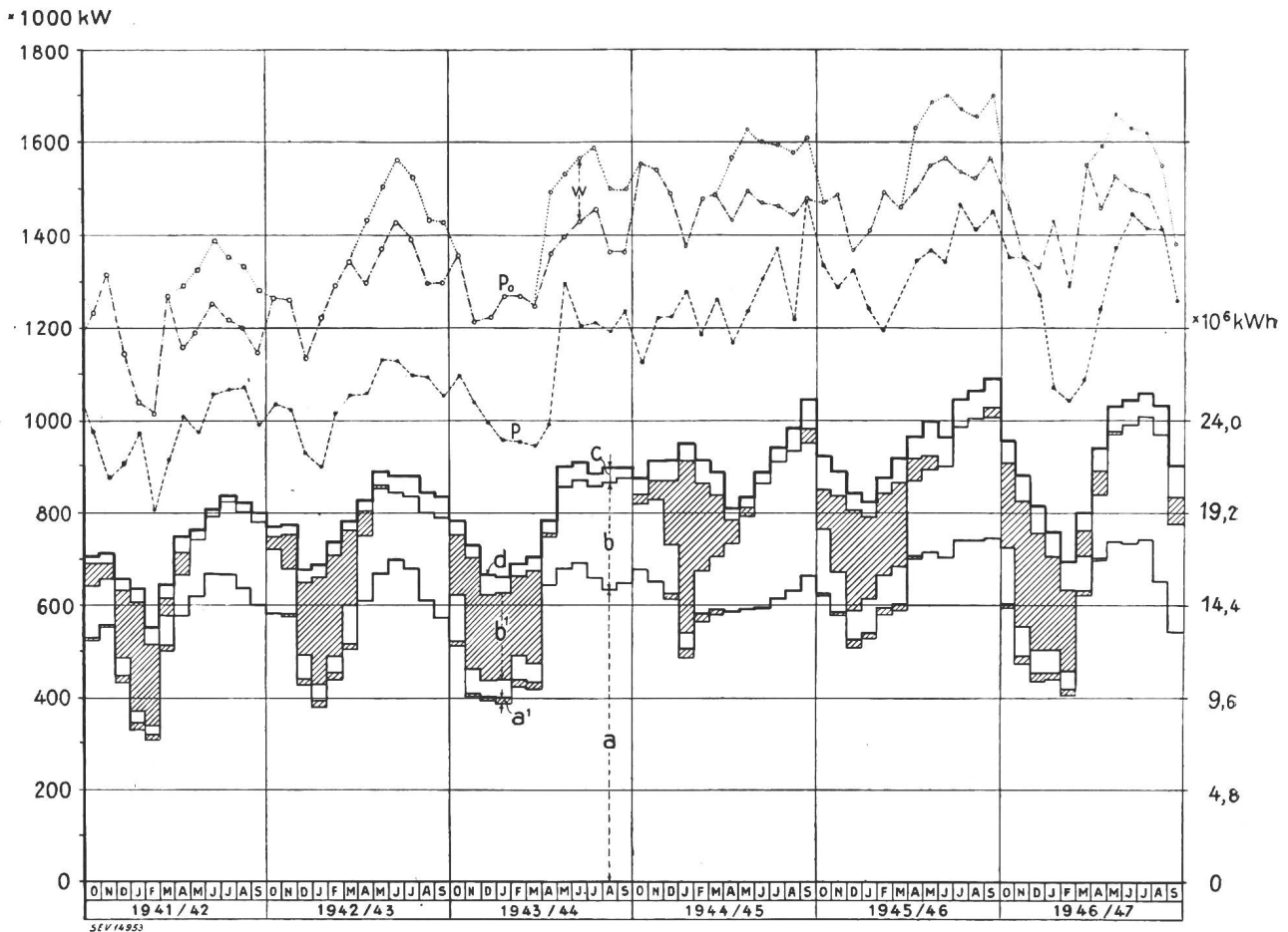
Fig. 3 Production mensuelle et puissances maxima
