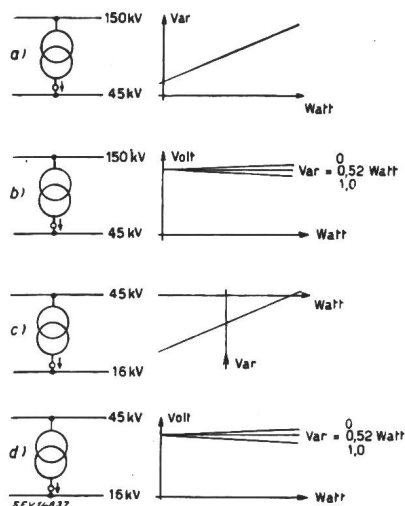
Fig. 1 Les quatre cas de réglage
