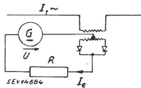
Fig. 4 Prinzipschema mit Gleichrichteranordnung in Mittelpunktschaltung I_1 ist in diesem Fall ein Wechselstrom
