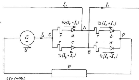
Fig. 5 Detailliertes Prinzipschema zur Erklärung der Wirkungsweise (Bezeichnungen wie in Fig. 1)
