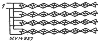
Fig. 37 Schematische Darstellung einer Richtantenne, bestehend aus 32 Dipolpaaren 1 Anschlussstelle für die Energiezuführung
