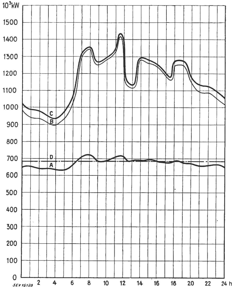
Diagramme de charge journalier du mercredi 18 février 1948
