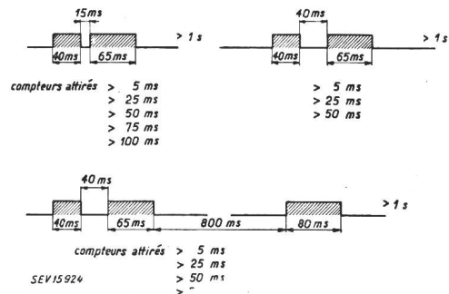
Fig. 2 Temps enregistrés par les compteurs pour diverses durées des signaux
