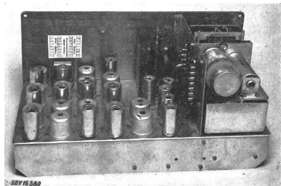
Fig. 8 Récepteur d'une station mobile
