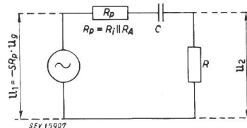
Fig. 15 Ersatzschema einer Stufe des Dreiphasen-RC-Generators der Fig. 14
