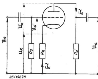
Fig. 6 Prinzipschema einer stromgegengekoppelten Verstärkerstufe
