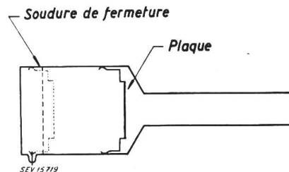
Fig. 4 Artifice pour protéger la plaque contre le traitement thermique
