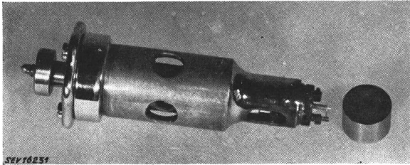
Fig. 21 Kathodeneinsatz
