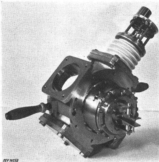
Fig. 22 Kathodenstrahlrohr
