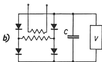
Schaltungen für Vollweggleichrichter
