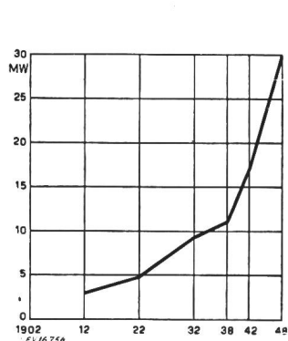
Fig. 14 Charge maximum annuelle du réseau de distribution en MW
