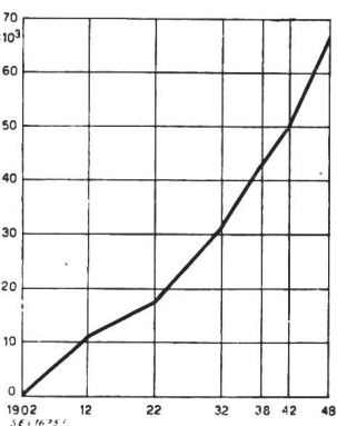
Fig. 13 Nombre de compteurs installés en milliers
