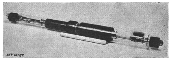
Fig. 9 Das «Graphophon», eine von der RCA entwickelte Bildspeicherröhre
