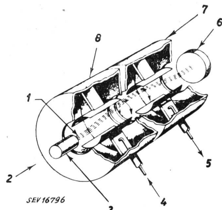
Fig. 16 Schnitt durch einen «Electron Coupler» 1 Elektronenstrahl 2 magnetisches Feld 3 Strahlkanone (Kathode) 4 Eingang 5 Ausgang 6 Kollektor 7 Ausgangs-Hohlraumresonator 8 Eingangs-Hohlraumresonator
