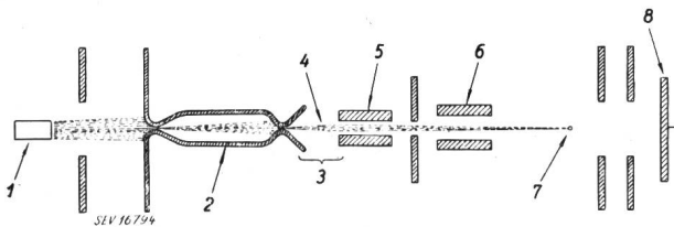
Fig. 14 Schematischer Querschnitt durch eine Mischröhre mit Doppelablenkung 1 Kathode 2 Blenden-System 3 Elektrostatische Linse 4 Elektronenstrahl 5 Signal-Ablenkplatten 6 Oszillator-Ablenkplatten 7 Abschattungsdraht von \frac{1}{10} mm Durchmesser 8 Anode
