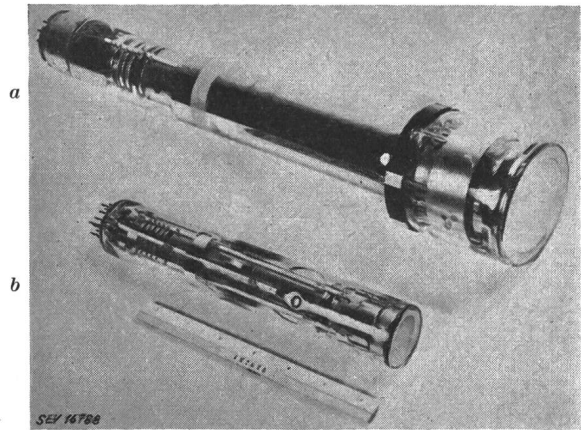
Fig. 8 Fernseh-Kameraröhren a RCA-2P23 Image-Orthicon-Röhre b «Mimo»-Kleinkameraröhre (RCA-2P22)
