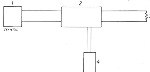
Fig. 15 Schaltschema des «Electron Couplers» 1 UHF-Leistungsgenerator 2 «Electron Coupler» 3 Belastung 4 Modulator
