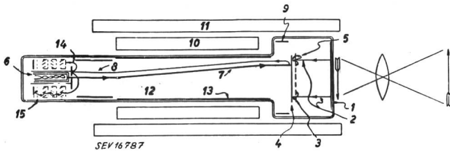
Fig. 7 Prinzipschema der RCA-Image-Orthicon-Fernsehaufnahmeröhre
