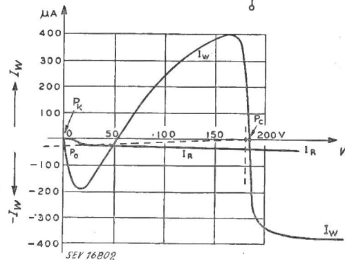
Fig. 22 Stromkurve einer Speicheröse des Selectrons 1 Schreibimpuls 2 Kathode 3 Kollektor 4 Öse 5 Schreibanode P_K Kathodenpotential P_C Kollektorpotential I Schreibstrom vom Ösenkopf I Lesestrom durch Ösenloch V Potential der Öse bezüglich der Kathode
