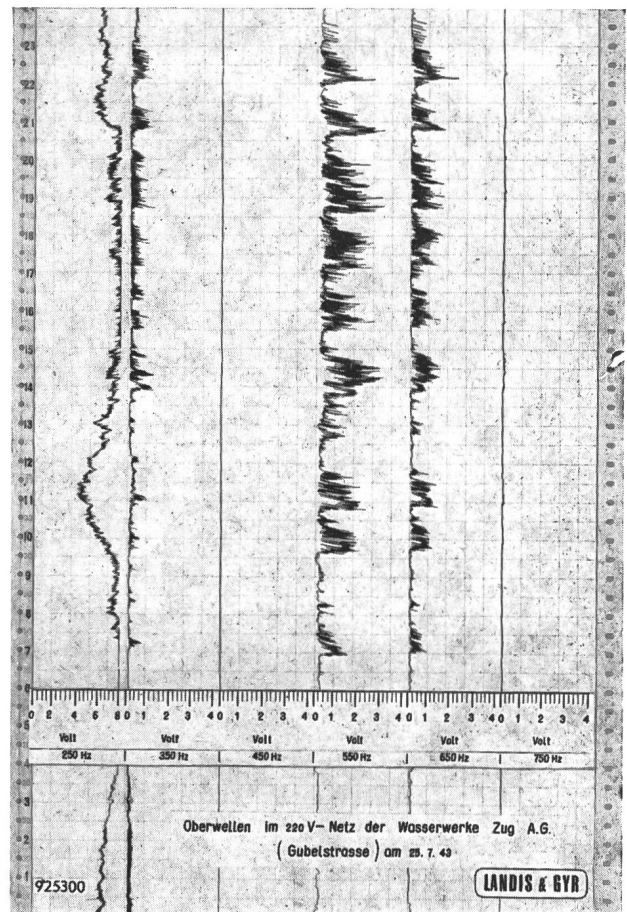
Fig. 2 Beispiel eines Registrierdiagramms der 5., 7., 9., 11., 13. und 15. Harmonischen
