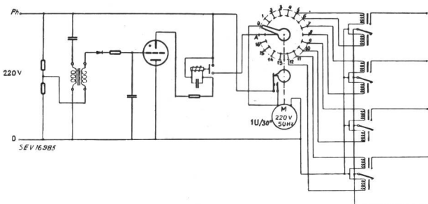
Fig. 1 Prinzipschema des Empfängers Von links nach rechts: Spannungsteiler, Resonanzkreis, Gleichrichter, Glimmröhre, Relais, Synchronwähler, Kippschalter
