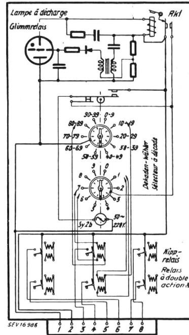
Fig. 2 Schema des Empfängers mit Dekadenwähler für 100 einfache Steuerbefehle Wahlkontakte 0...9: Einer-Reihe Wahlkontakte 00...99: Zehner-Reihe
