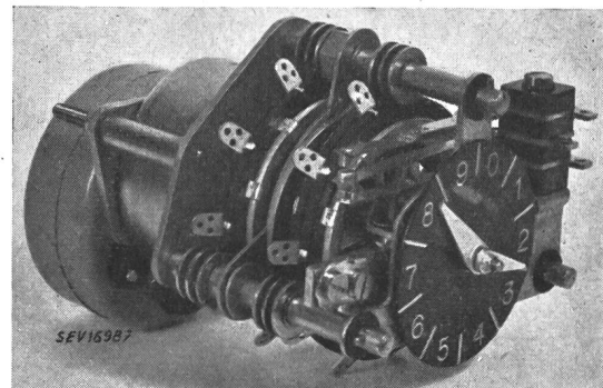
Fig. 3 Dekadenwähler für 100 einfache Steuerbefehle mit Synchronmotor, gekapseltem Getriebe, zwei Kontaktreihen zu je 10 Kontakten und Stellungszeiger
